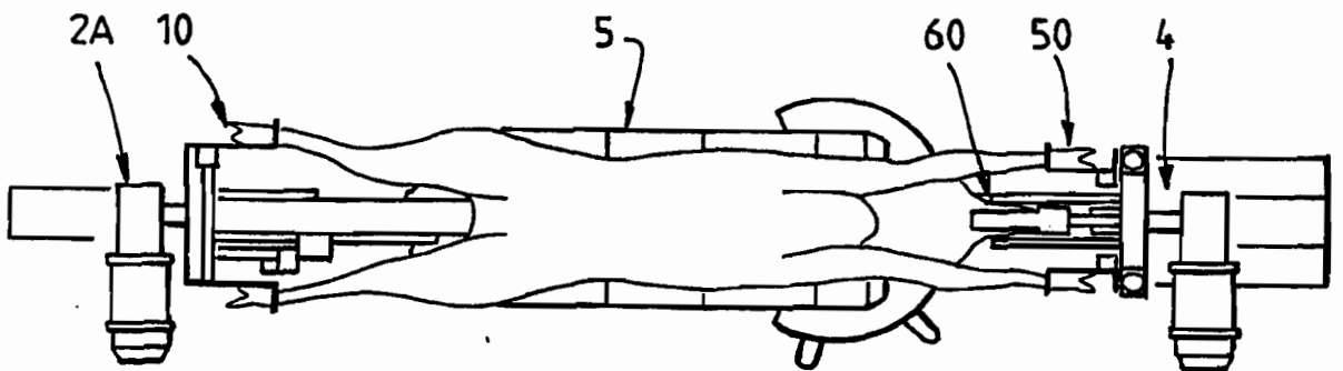
FIG. 24. Shearing position 11
